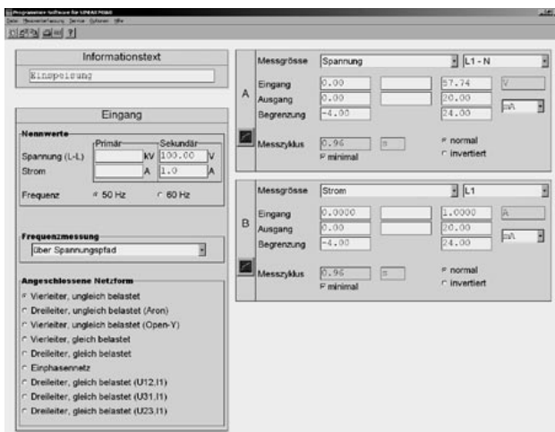
Bild 5. Darstellung aller Programmierparameter im Hauptmenü.
