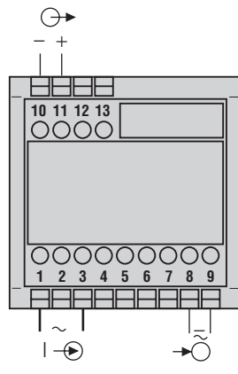
Bild 3. Für Messung mit zweitem (größerem) Messbereich, Hilfsenergie-Anschluss an Klemmen 8 und 9.
