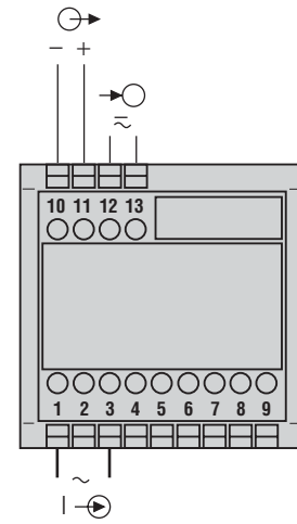
Bild 5. Für Messung mit zweitem (größerem) Messbereich, Hilfsenergie-Anschluss auf Niederspannungsseite an Klemmen 12 und 13.
