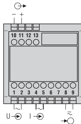
Fig. 2. Power supply to terminals 8 und 9.
