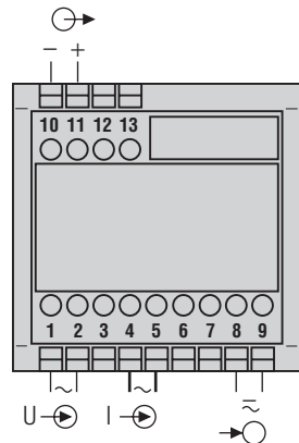
Fig. 2. Alimentation auxiliaire sur bornes 8 et 9.
