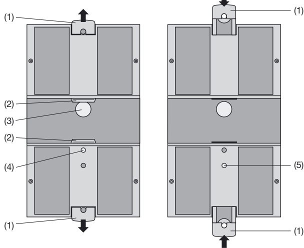
Bild 5. Geräteboden.
