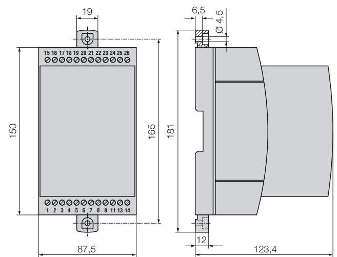
Fig. 15. SINEAX DME en boîtier T24 avec languettes extraites pour montage mural direct.
