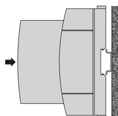
Fig. 5. Montage sur rail «à chapeau» 35 × 15 ou 35 × 7,5 mm.
