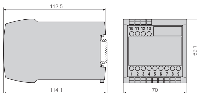
Fig. 4. Boîtier P13/70 encliqueté sur rail «à chapeau» (35 × 15 mm ou 35 × 7,5 mm, selon EN 50 022).
