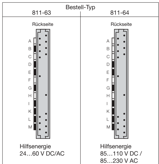
Bild 4. Codierung des Steck-Moduls SIRAX B 811 in [EEx ia] IIC-Ausführung .
