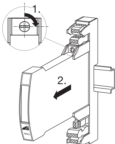
Bild 15. Steck-Modul herausziehen.
