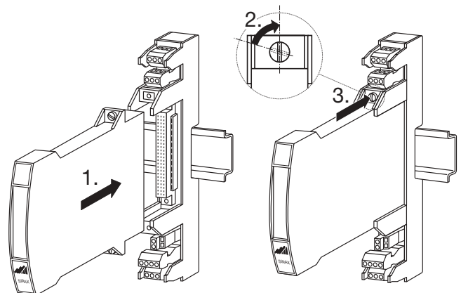
Bild 14. Steck-Modul aufstecken.
