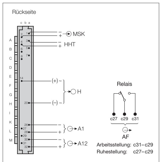
Bild 6. Steckerbelegung. Sicht auf die Rückseite des SIRAX B 811.
