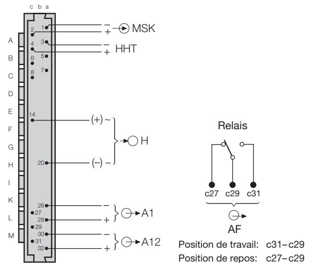
Fig. 6. Plan des fiches. Vue depuis l'arrière du SIRAX B 811.
