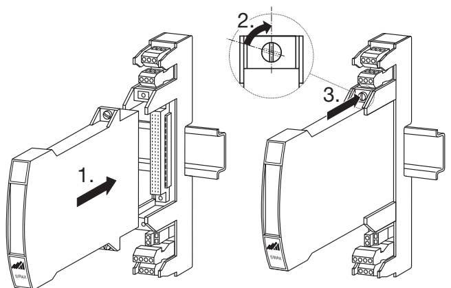
Fig. 14. Enficher le module embrochable.
