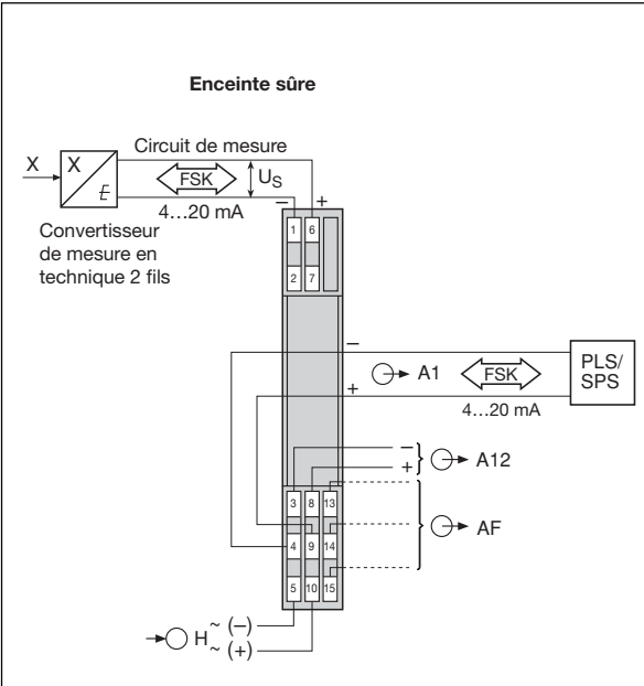
Fig. 12. SINEAX Type 811-1..2 .... , circuit de mesure et sortie non en sécurité, intrinsèque, tension d'alimentation U_s 24 V CC, avec transmission de la communication. Automate programmable raccordé sur sortie A1.
