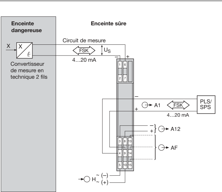
Fig. 13. SINEAX Type 811-1..2 .... , circuit de mesure en sécurité intrinsèque, tension d'alimentation U_s 16,4 V CC, avec transmission de la communication. Automate programmable raccordé sur sortie A1.
