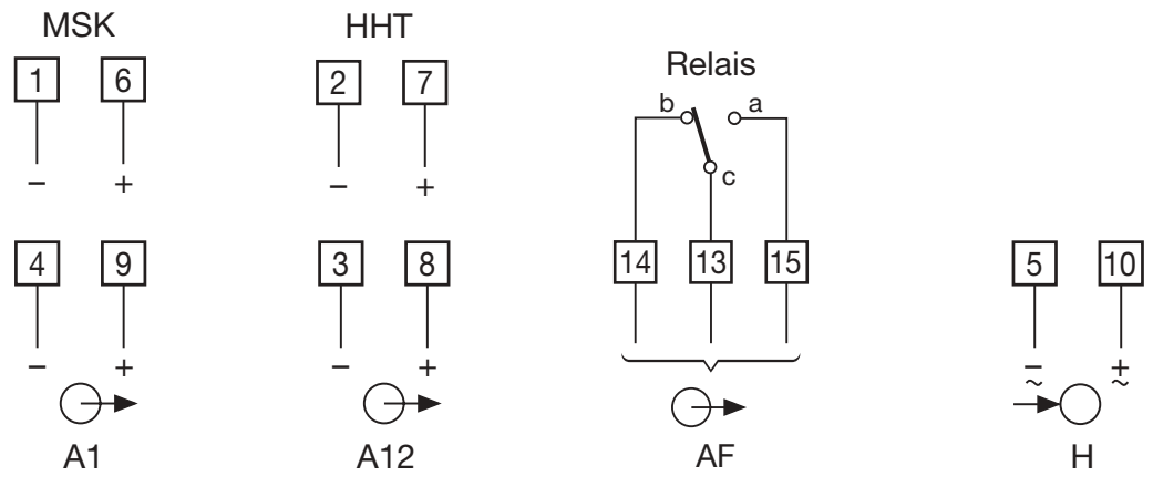
Ohne Klarsicht-abdeckung
